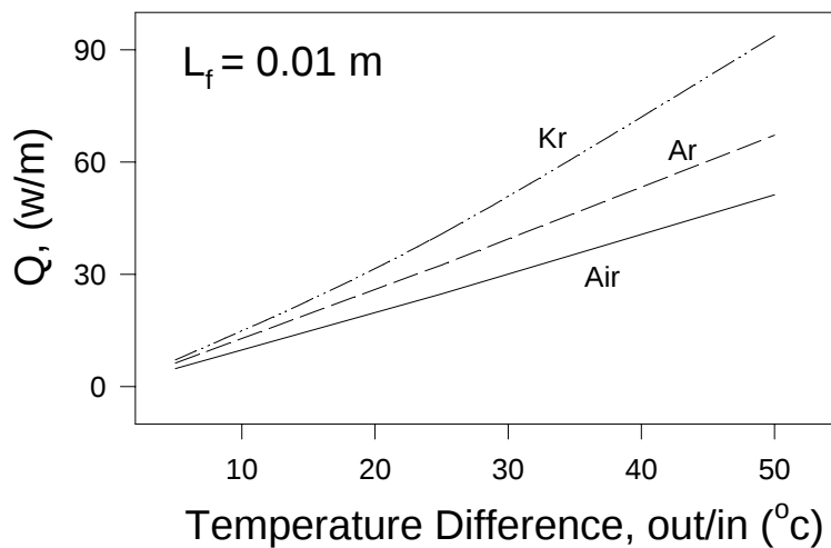
شکل ۶- تغییرات اتلافات حرارتی با اختلاف دمای دو طرف پنجره برای گازهای مختلف با در نظر گرفتن انتقال حرارت جابه جایی آزاد
