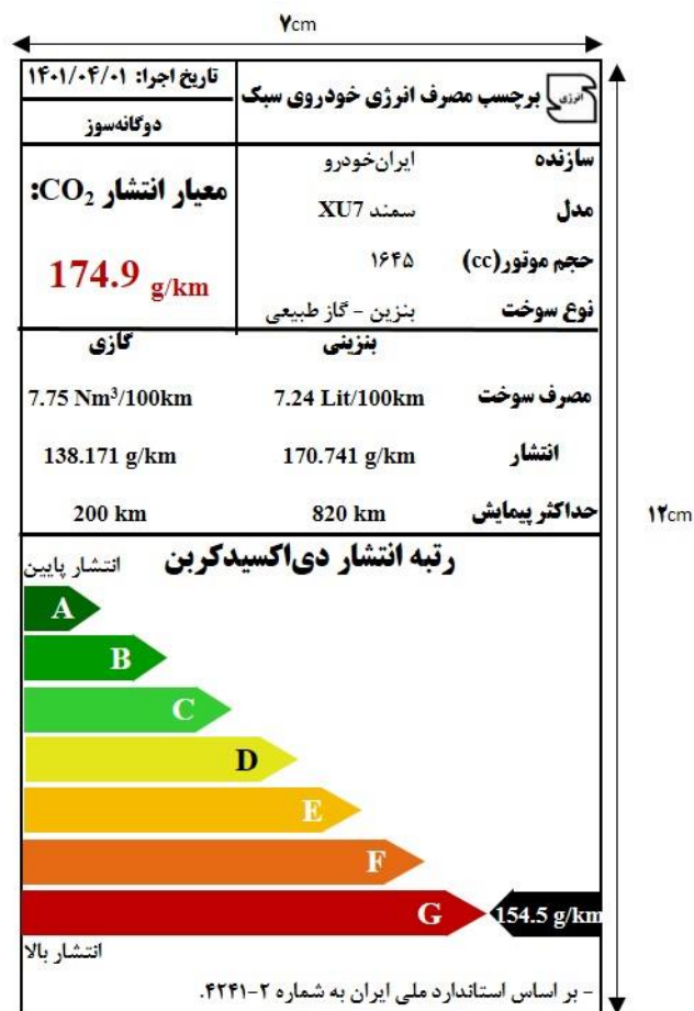
شکل ۳- نمونه برچسب خودروهای دوگانه‌سوز بنزین-گاز (LPG یا CNG) به همراه ابعاد
